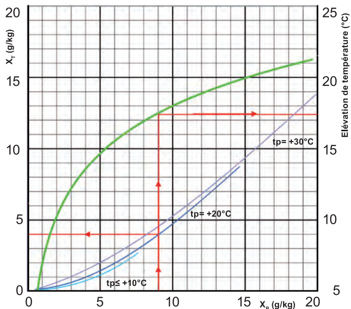
Diagramme de capacité pour un débit d'air sec de 2300 m 3 /h
