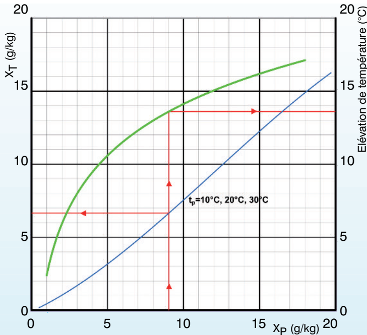
DIAGRAMME DE CAPACITÉ débit d'air sec de 210 m 3 /h
