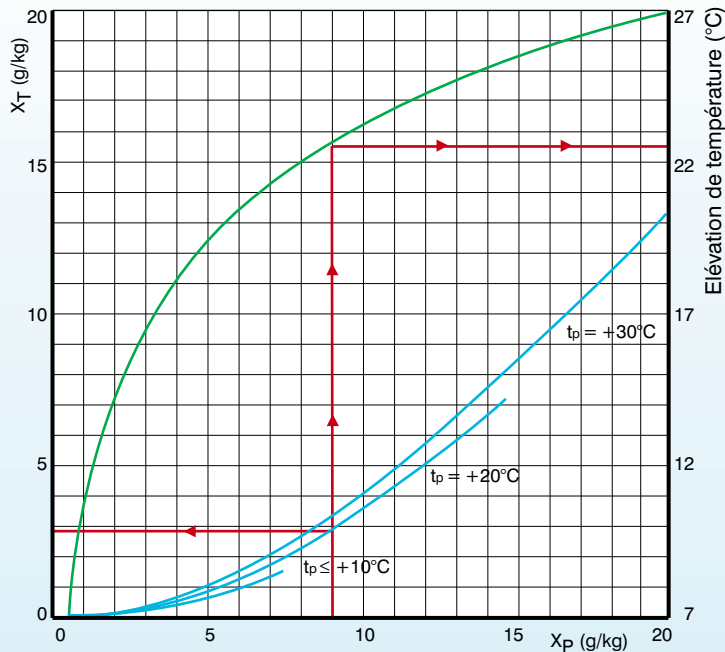
DIAGRAMME DE CAPACITÉ débit d'air sec de 1000 m 3 /h
